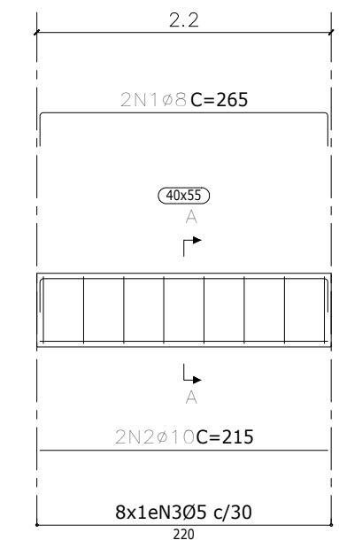
V 101 V 102
