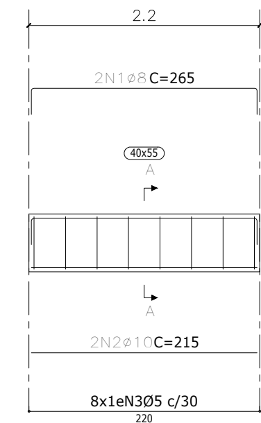
V 101 V 102
